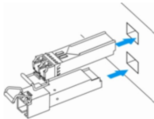
Рисунок 62 – Установка SFP-трансиверов
