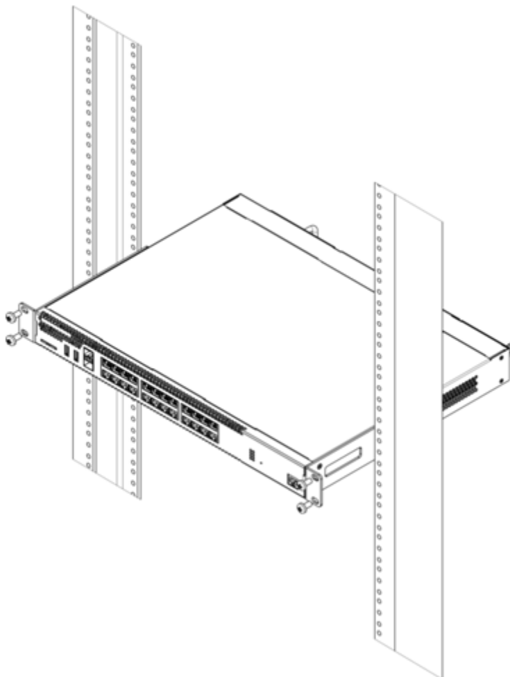
Рисунок 59 – Установка устройства в стойку
