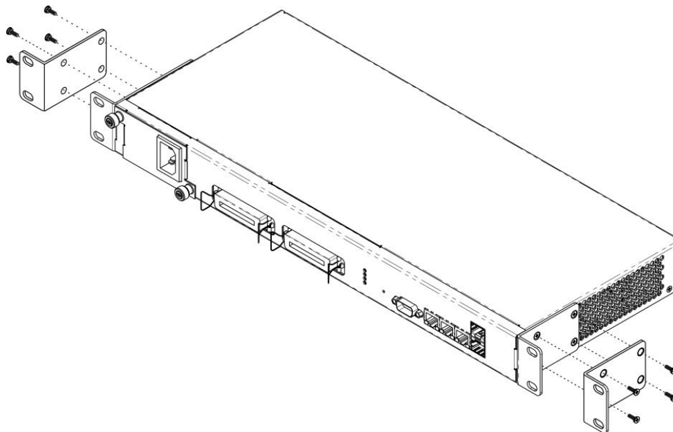
Рисунок 11 – Крепление кронштейнов
