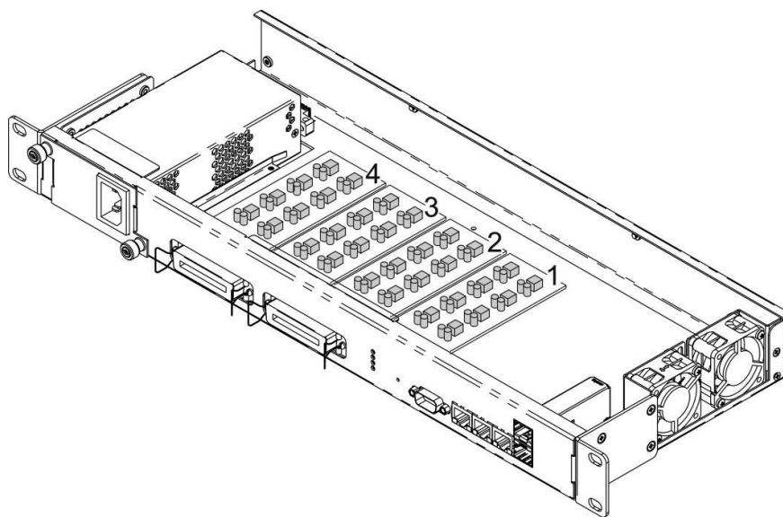
Рисунок 14 – Расположение submodule в TAU-32M.IP
