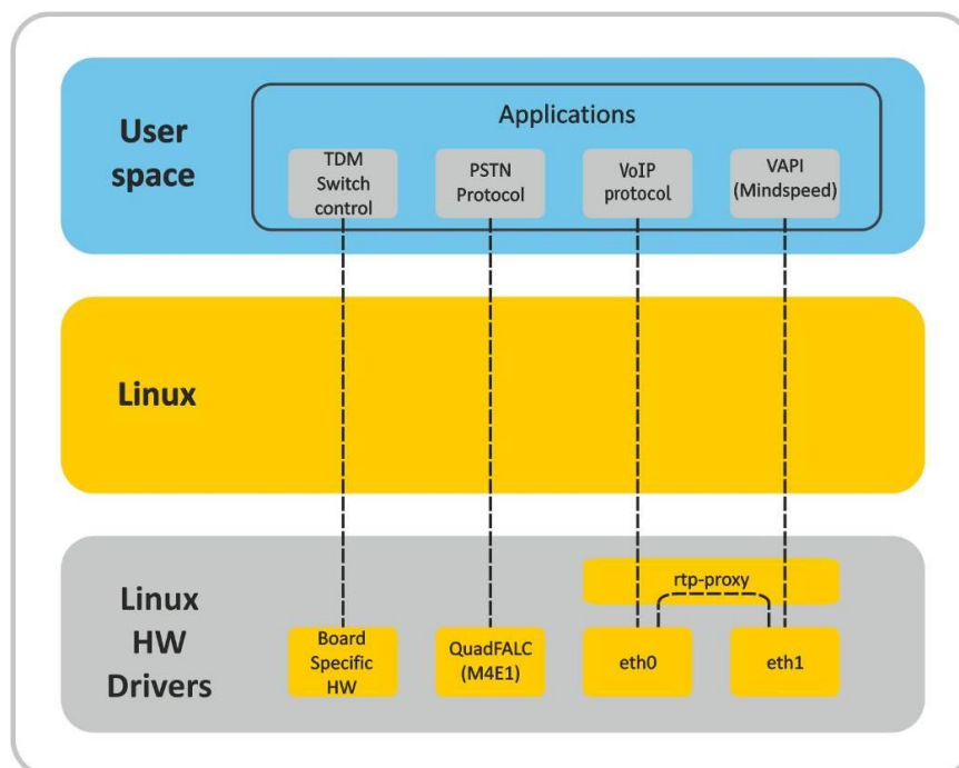
Рисунок 6 – Структура программного обеспечения SMG
