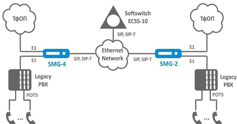
Рисунок 3 – Сопряжение сигнализации и медиапотокков TDM- и VoIP-сетей
