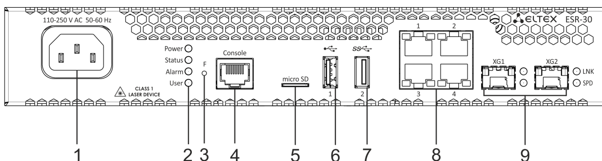
Рисунок 36 – Передняя панель ESR-30
