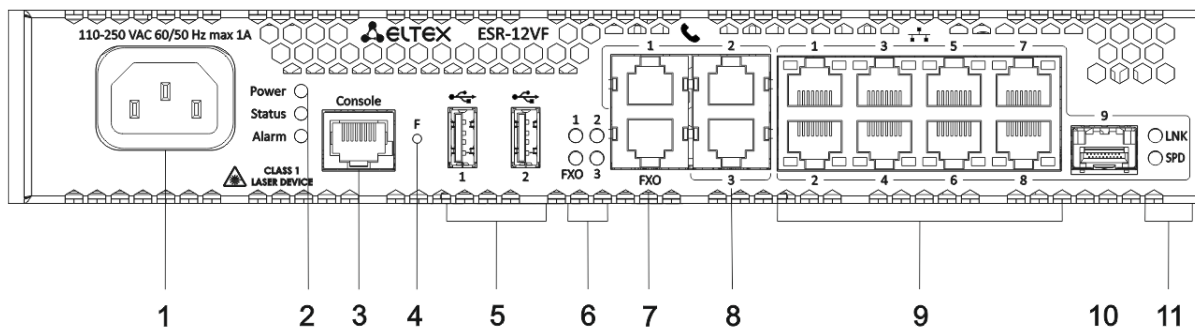
Рисунок 47 – Передняя панель ESR-14VF, ESR-12VF
