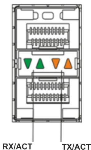
Рисунок 61 – Расположение индикаторов оптических интерфейсов
