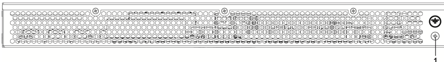
Рисунок 33 – Задняя панель ESR-21
