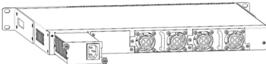
Рисунок 73 – Установка модулей питания
