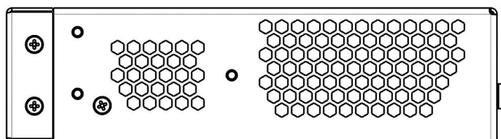
Рисунок 46 – Правая боковая панель ESR-15R
