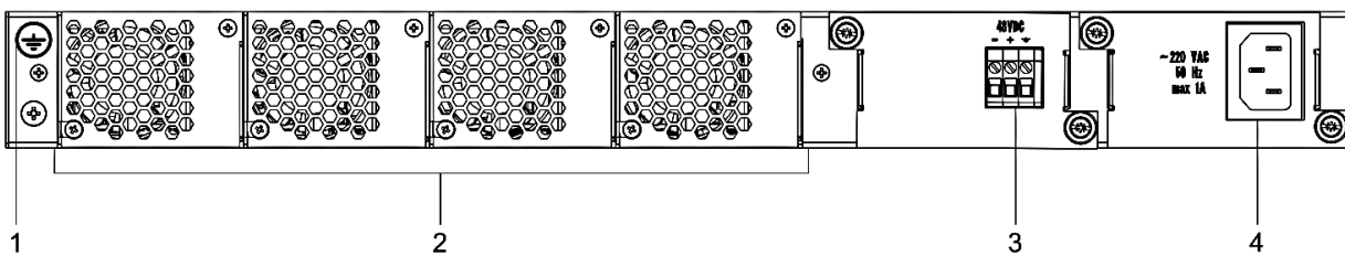
Рисунок 28 — Задняя панель MES3324F, MES3348F, MES3324
