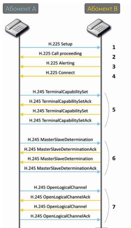
Рисунок 20 – Алгоритм вызова по протоколу H.323
