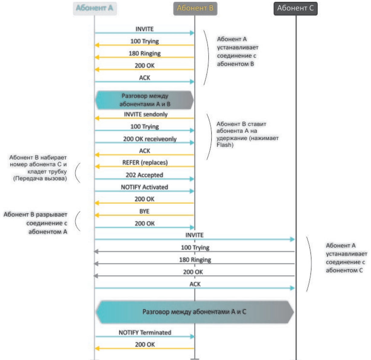
Рисунок 12 – Алгоритм выполнения услуги «Перевод вызова без сопровождения» («Unattended calltransfer») абонентом «В» по протоколу SIP
